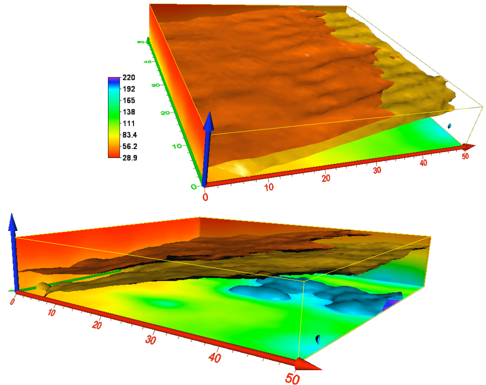
Рис. 3. Распределение УЭС под стройплощадкой
